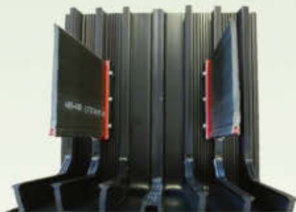
Abdichtungssysteme gegen drückendes Wasser - Gleitlager
